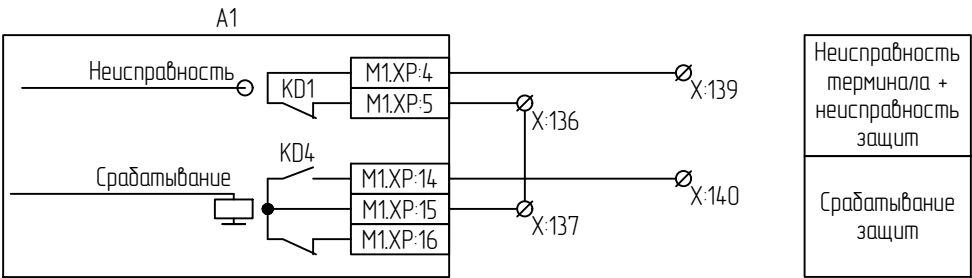
Цепи РАС
