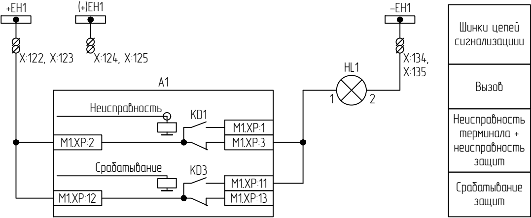
Цепи сигнализации
