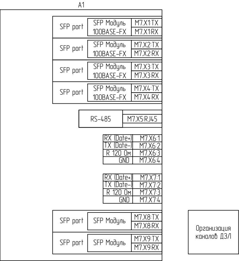
Цепи связи терминала
